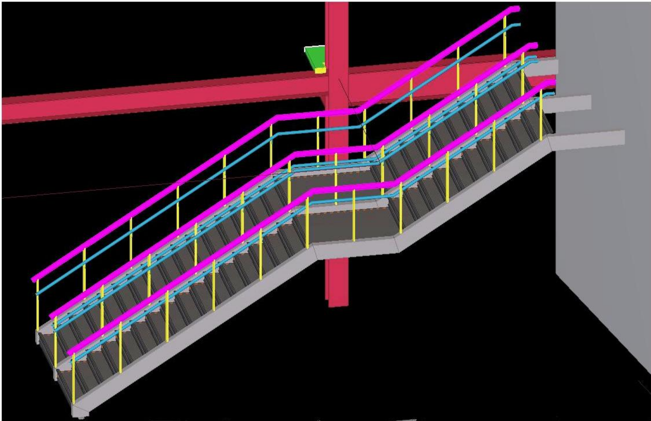
STAIR - 5
